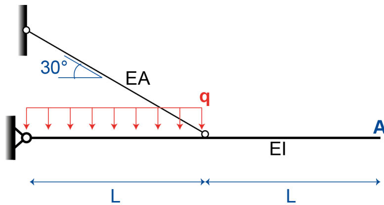
Figure 1 – Poutre suspendue à un câble
